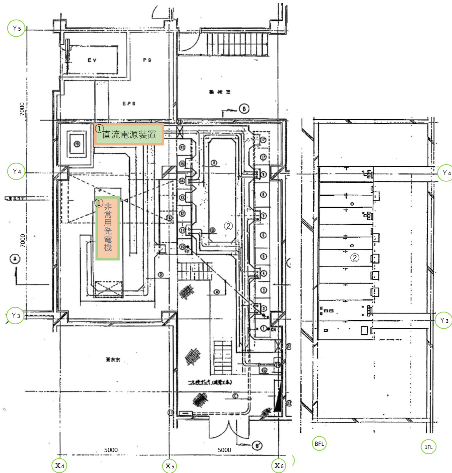
電気室平面図
