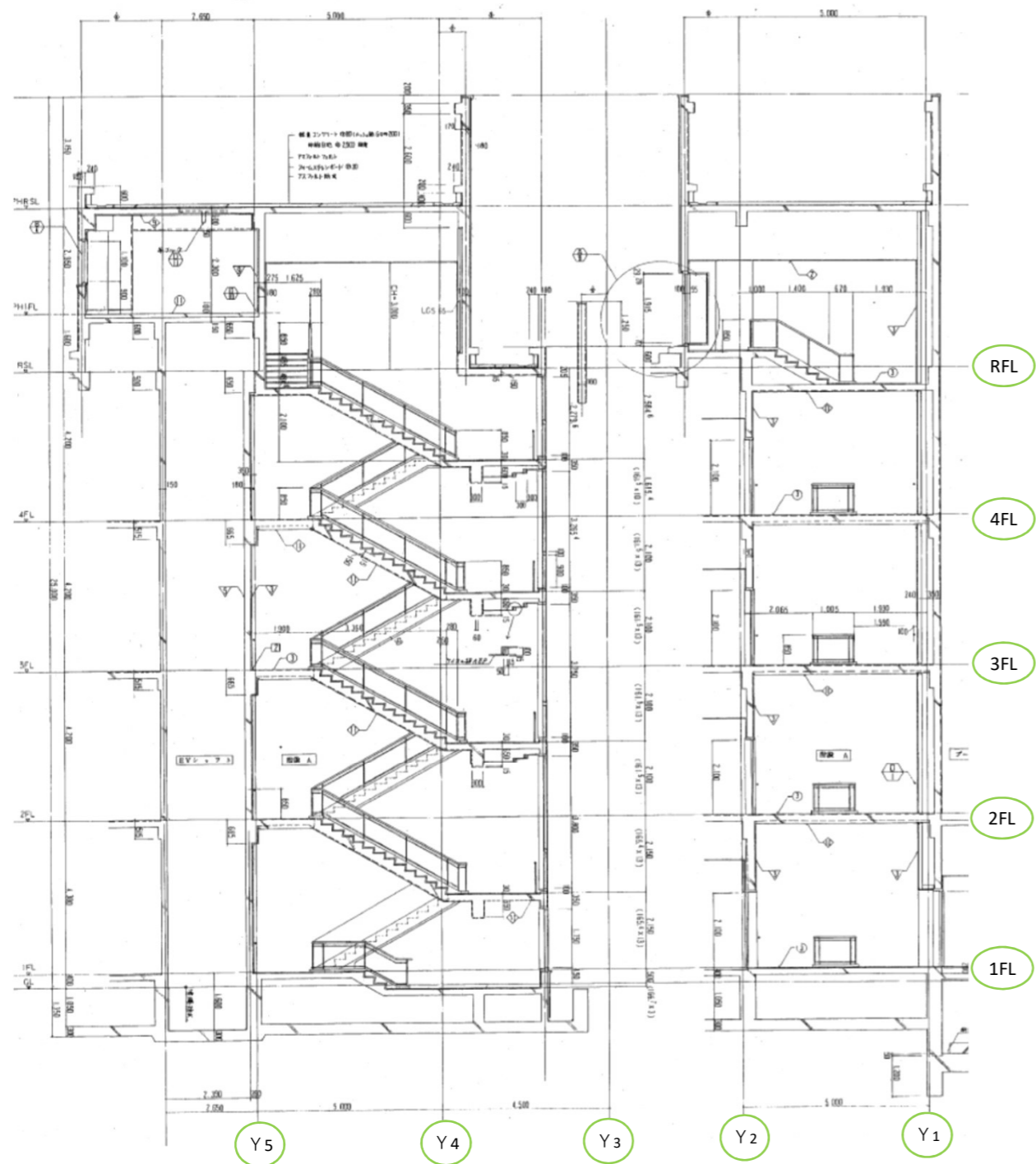
階段断面図
