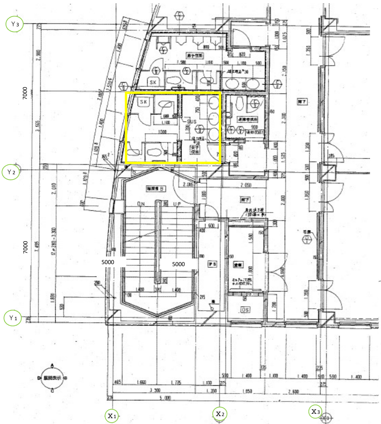
3階トイレ平面図
