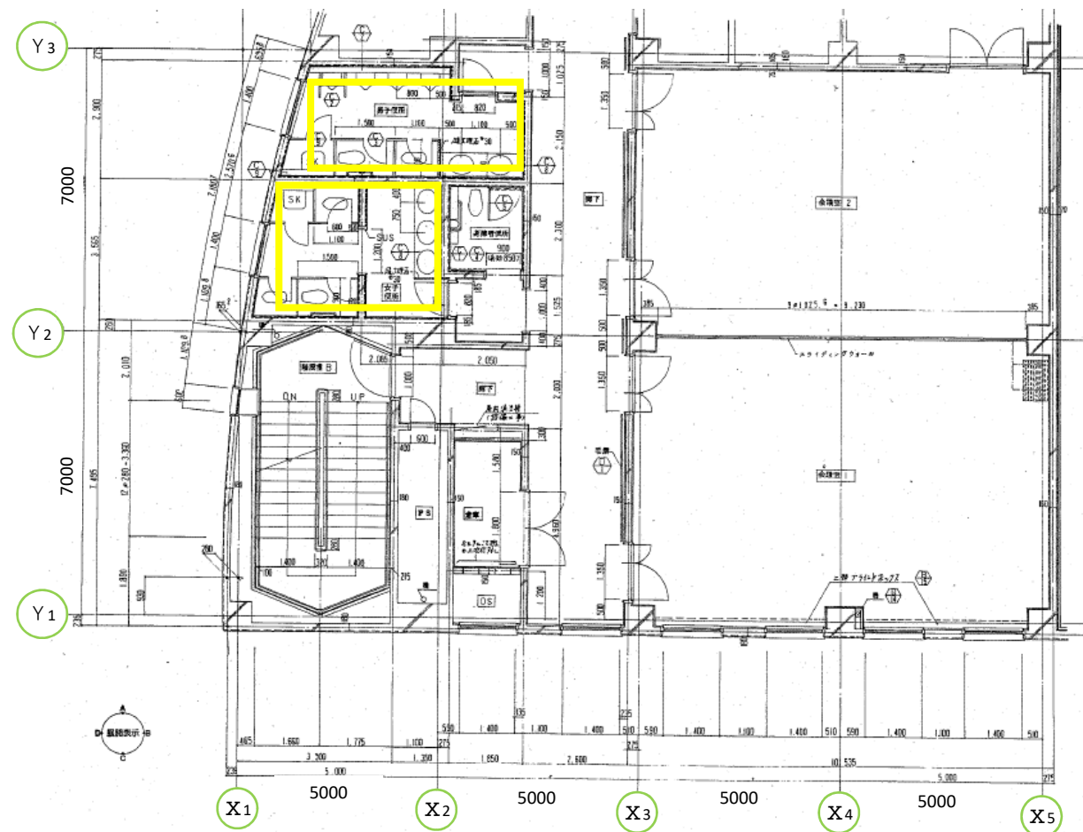
3階トイレ平面図
