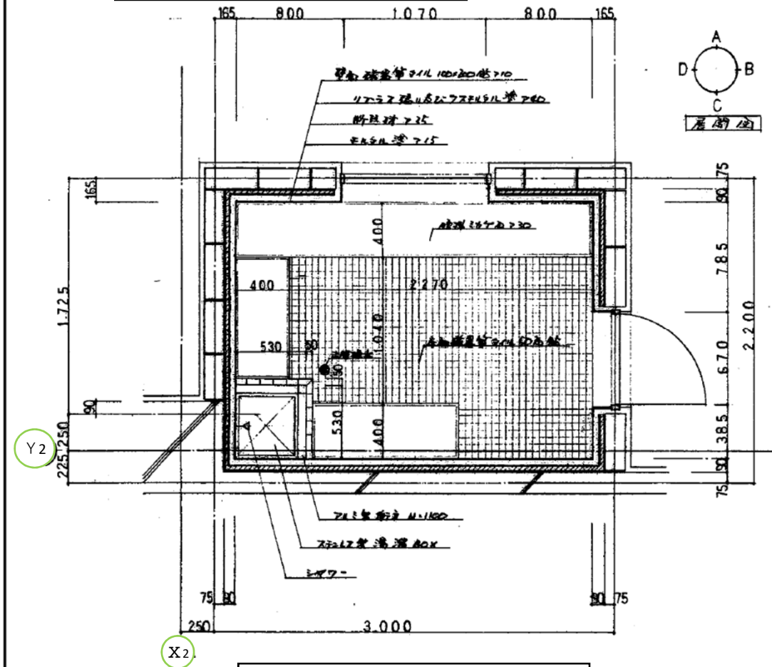
女子サウナ室平面図
