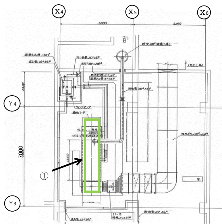
電気室平面図
