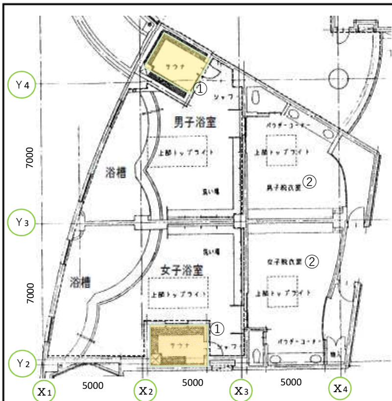
4階風呂まわり平面図
