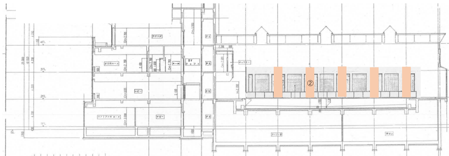
Y4断面図
