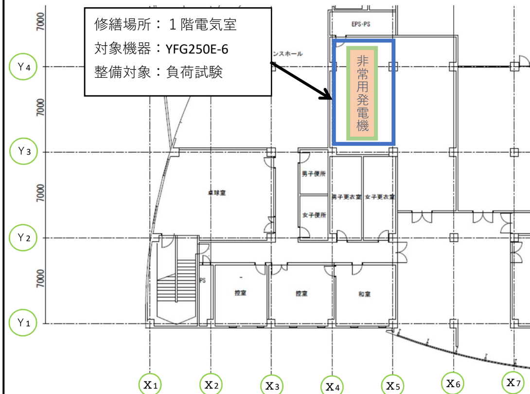
1階平面図
