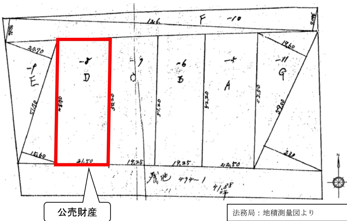
地積測量図
