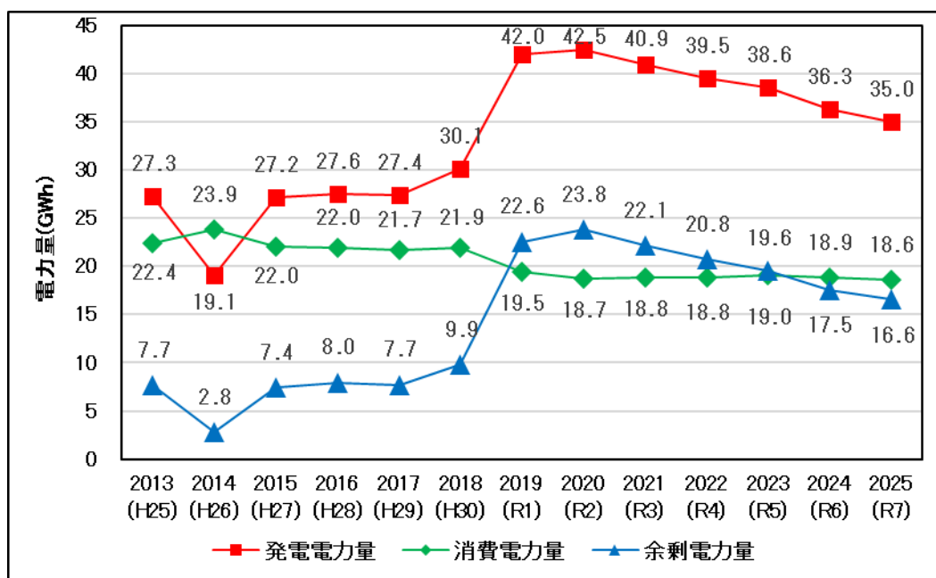
図2-6 エネルギーセンターにおける廃棄物発電の発電電力量等の推移
