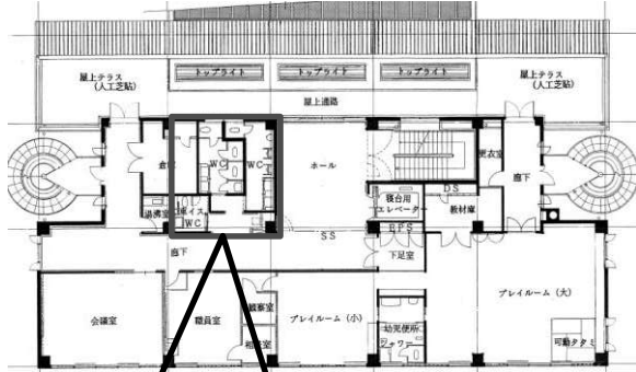
3階平面図
