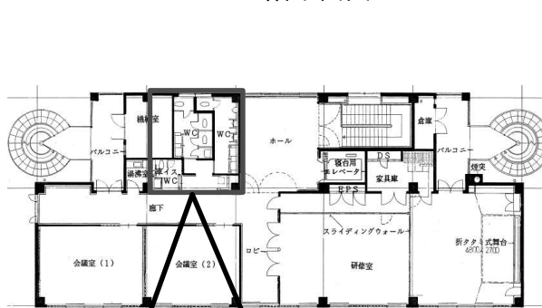
4階平面図
