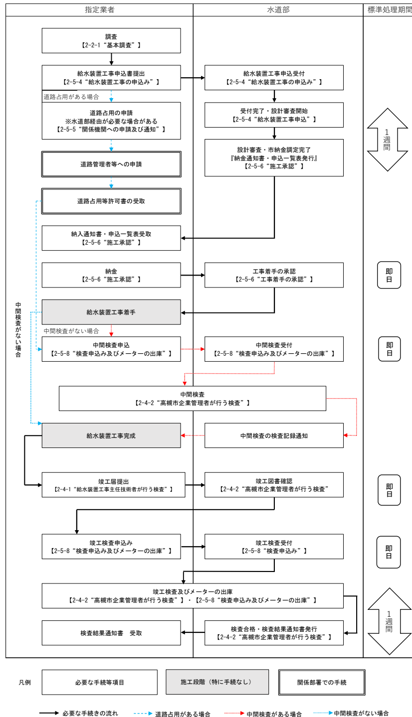
図-2.5.2.1 標準的な給水装置工事のフロー
