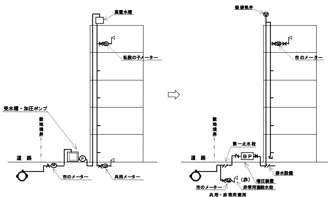
図-2.2.16.2 高置水槽式から直結増圧式への切替工事例（切替前／切替後）
