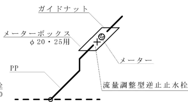
図-2.2.10.3 流量調整型逆止止水栓
