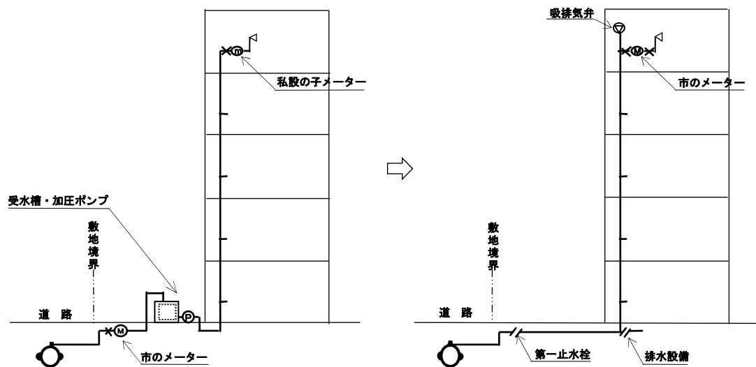
図-2.2.16.1 受水槽式（加圧式）から直結直圧式への切替工事例（切替前／切替後）
