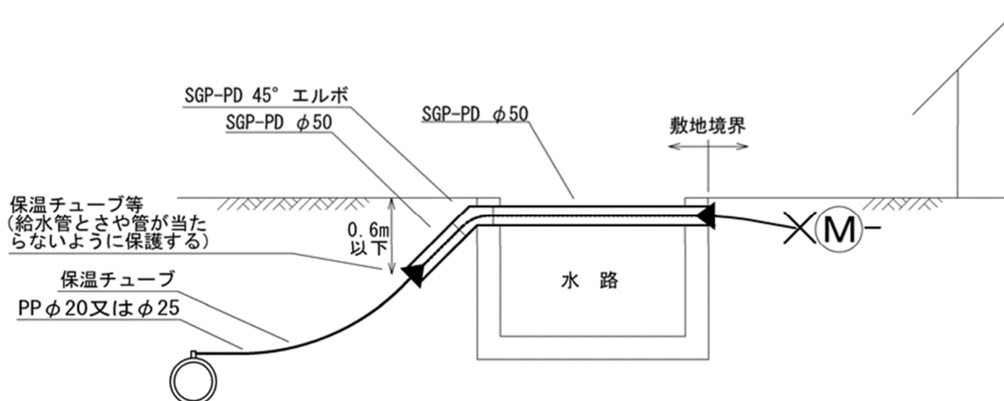
※ 埋設が浅くなる箇所は、道路表面に標示するよう努めること 図-2.2.8.3 ポリエチレン管による水路添架の施工例（下越しが困難な場合）
