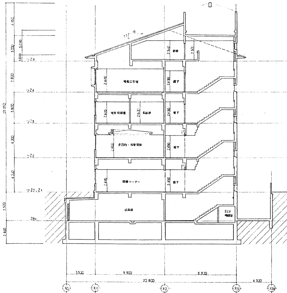
B-B 断面図 1/100
