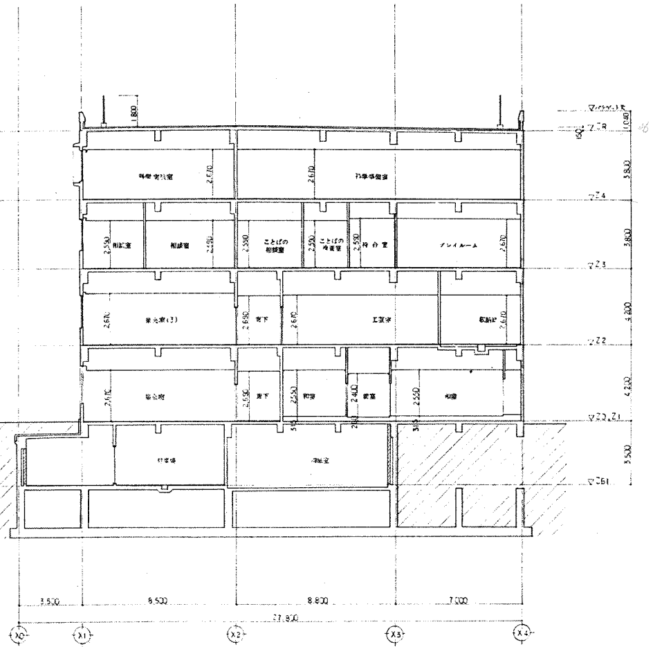
C-C 断面図 1/100
