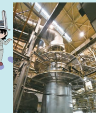
洗浄塔。硫酸酸化物や塩化水素などを除去
