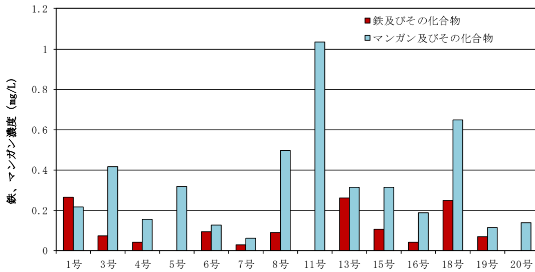
図1 大冠浄水場各取水井の鉄、マンガン濃度(令和6年度平均)
