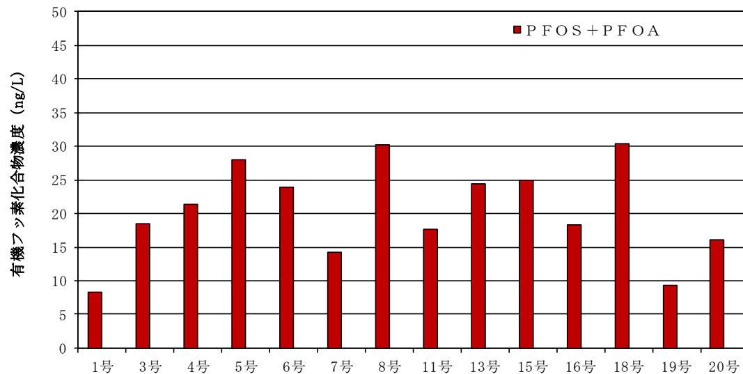
図3 大冠浄水場各取水井の有機フッ素化合物濃度(令和6年度平均)
