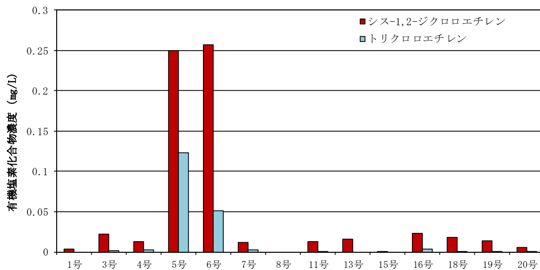
図2 大冠浄水場各取水井の有機塩素化合物濃度(令和6年度平均)
