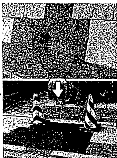
紺屋町 ●陥没した歩道整備
