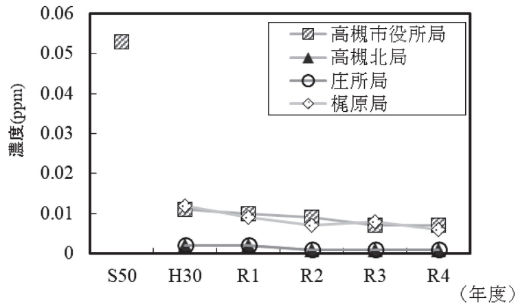
図5-5 一酸化窒素濃度の経年変化 (年平均値)
