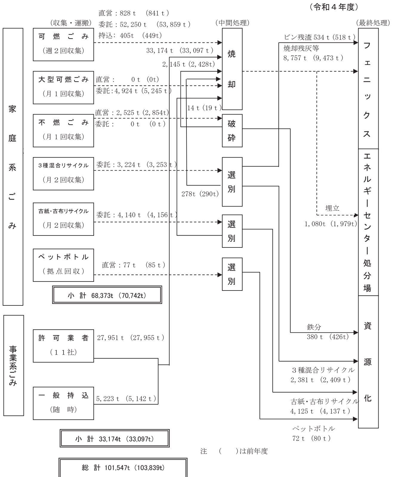
図7-2 ごみ処理フロー
