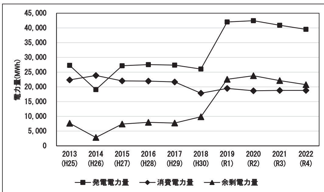
図2-6 エネルギーセンターにおける廃棄物発電の発電電力量等の推移
