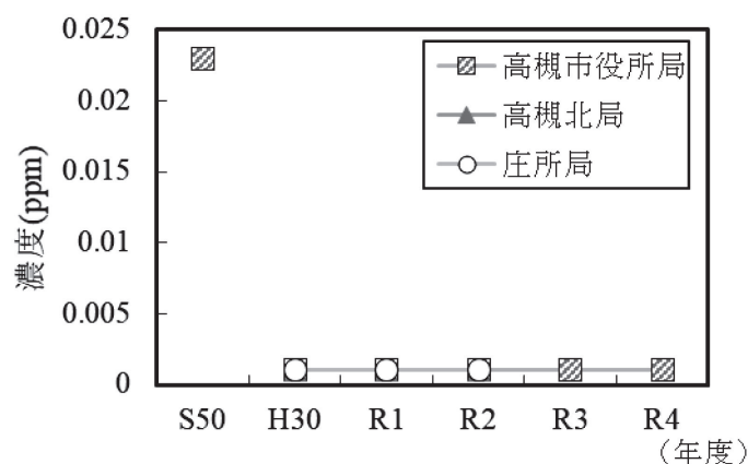
図 5 - 2 二酸化硫黄濃度の経年変化（年平均値）
