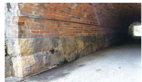
JR京都線のトンネル 朝日町の下阪谷架道拱梁、下部には石垣石がはまっている
