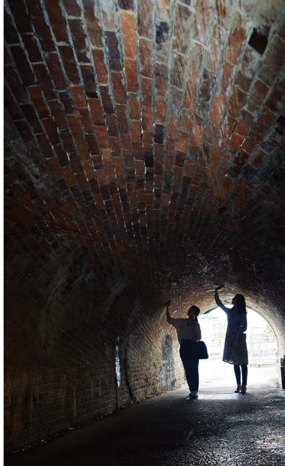
梶原のトンネルは、南側がねじりまんぼ、北側は当時近代的だったコンクリートという2つの顔を持つ。明治初期に鉄道が開業してから100年以上も利用されている。全国のねじりまんぼを巡るマニアもいるのだそう
