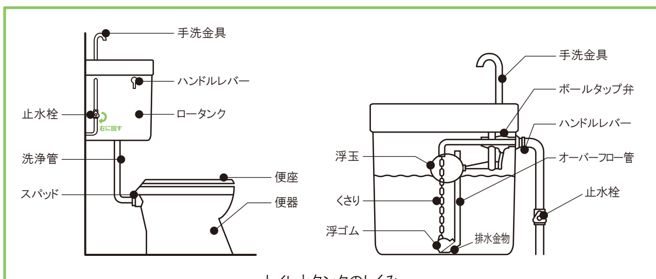
トイレとタンクのしくみ
