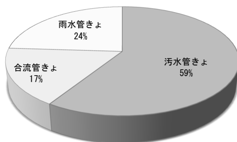
図 1-8 管きよ施設の内訳
