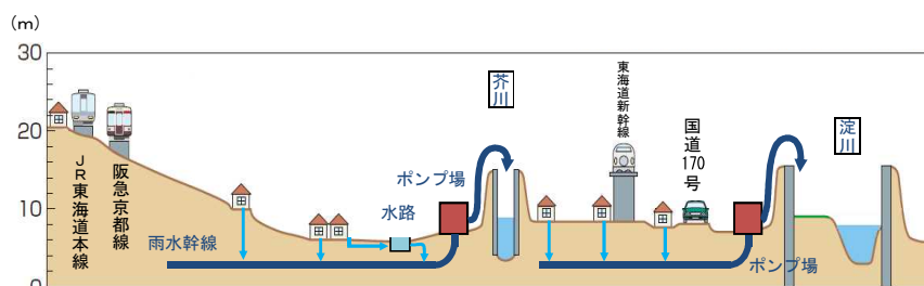
図1-1 模式断面図
