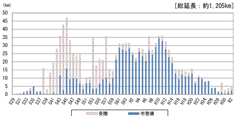
図 1-7 年度別の整備延長
