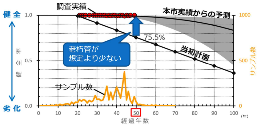
図3-1 健全度予測（緊急度Ⅰ）
