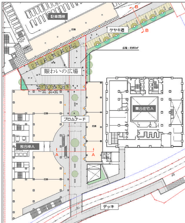
■デッキ平面図 (Aエリア一部)
